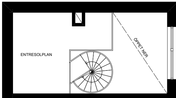
Plan 2 entresol
