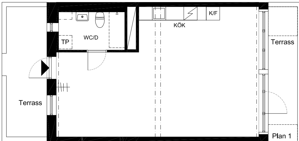
Plan 2 (primärbalkar för möjligt loft)
